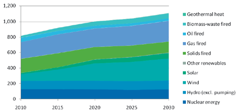
Previsión de la capacidad de generación de energía en Europa en 2030 (GW). Fuente: EU energy trends to 2030
