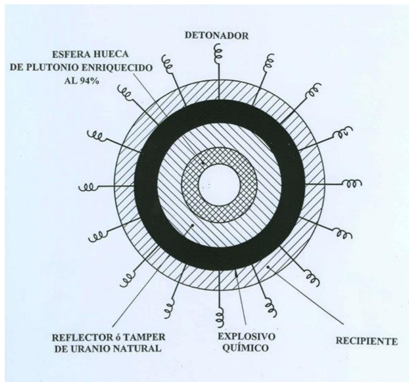
Figura 2.- Esquema del método de la implosión empleado en las bombas atómicas de plutonio
