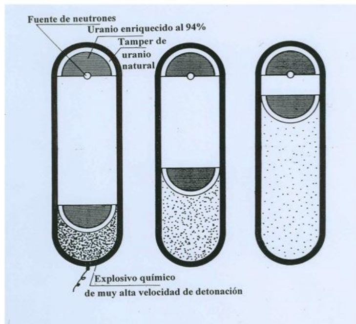
Figura 1.- Esquema del método del proyectil
